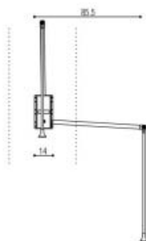
side view - solution 2 側面図2 fixed to the sides center キャビネット側板中央に取り付ける
