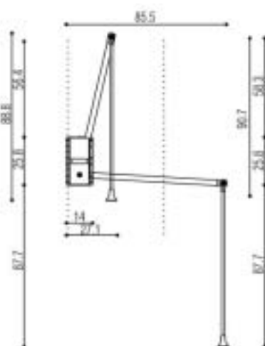
side view - solution 1 側面図1 with inclination the device キャビネット側板奥に取り付ける
