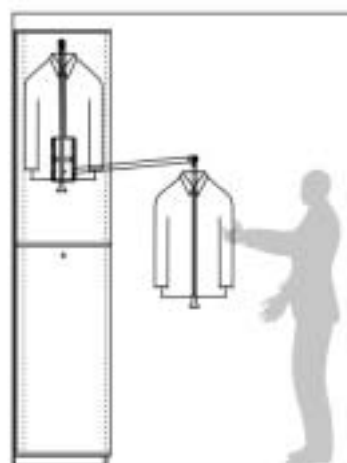
side view - solution 2 側面図2 fixed to the sides center キャビネット側板中央に取り付ける
